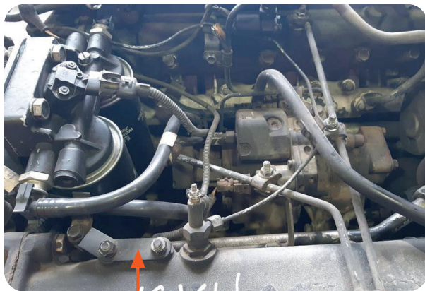
Кронштейн трубки низкого давления с ТНВД BOSCH
