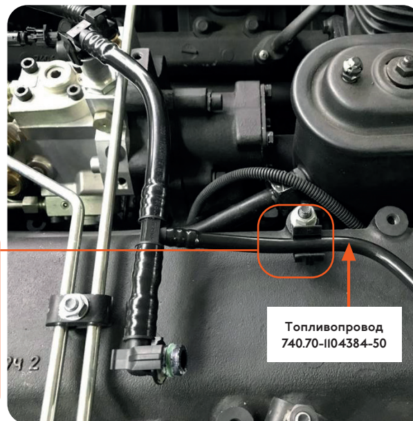
Топливопровод 740.70-1104384-50
