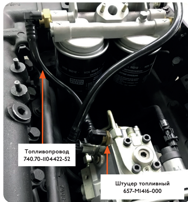
Топливопровод 740.70-1104422-52
