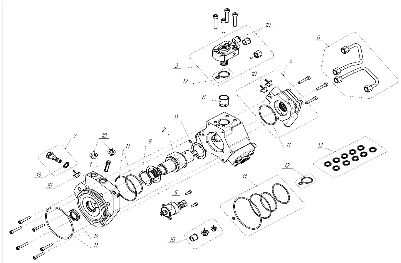
Рисунок 1 – Ремонтные комплекты и запасные части ТНВД А-08-004-00-00-01
