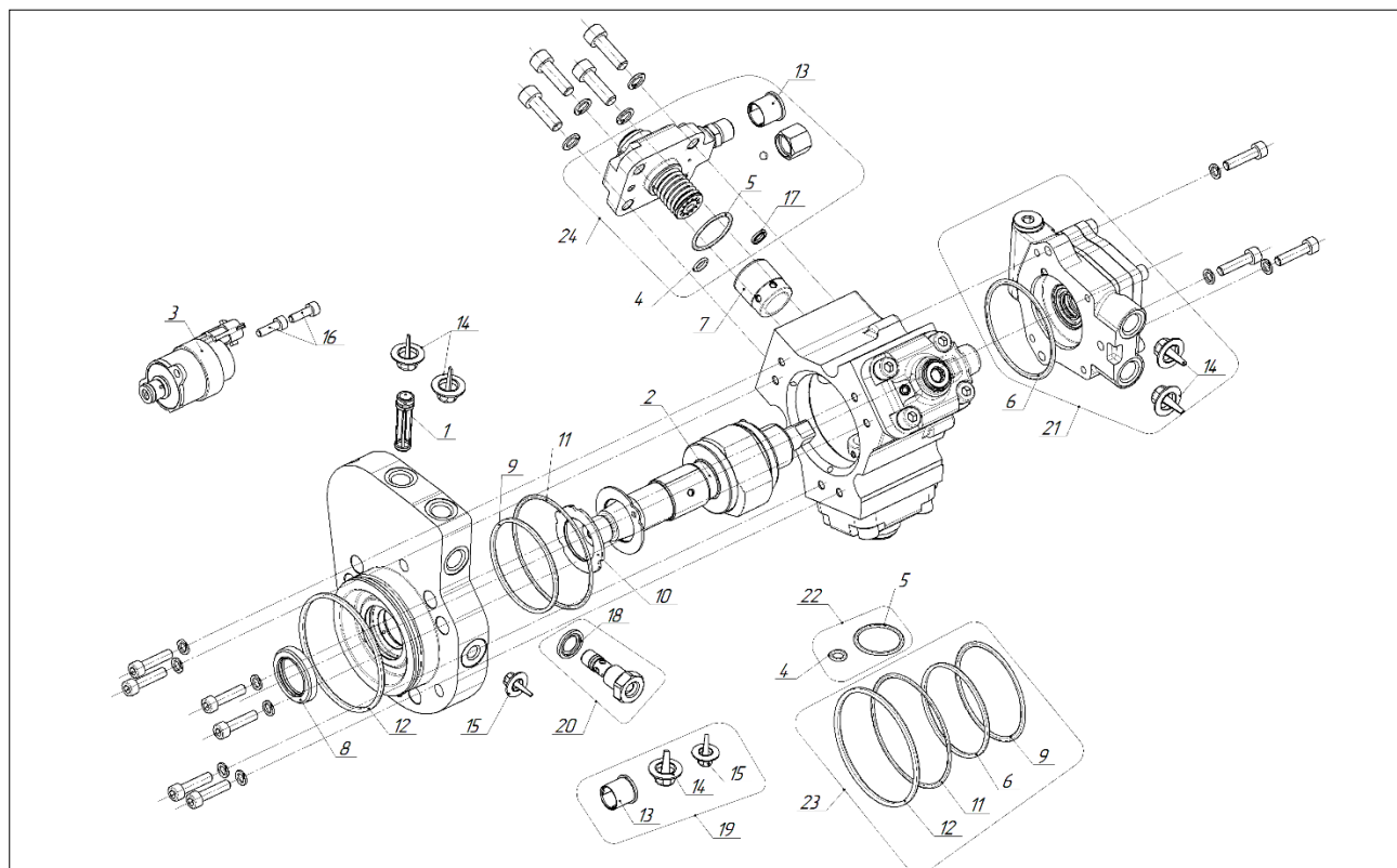
Рисунок 2 – Запасные части и комплекты для ремонта ТНВД А-08-013-00-00-10.
