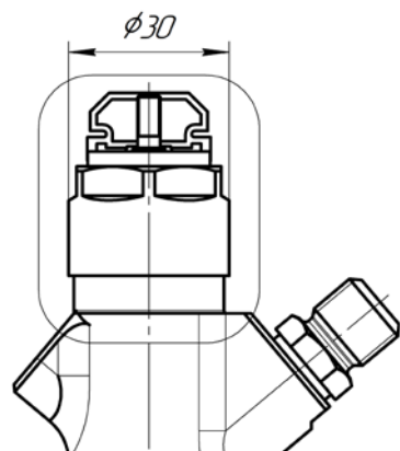
Рисунок 4. Инжектор А-04-017
