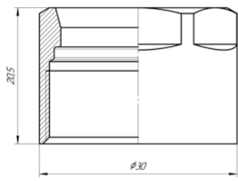
Рисунок 2. Гайка электромагнита.
