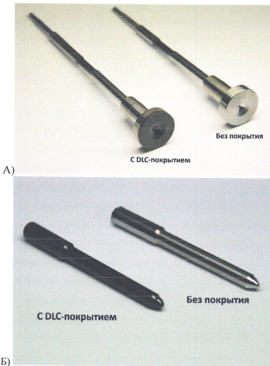
Рисунок 1– Комплектующие CR производства АЗПИ (А– клапан управляющий, Б – игла распылителя)
