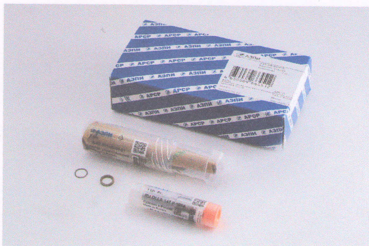
Рисунок 1 – Комплект запасных частей для ремонта инжекторов Common Rail
