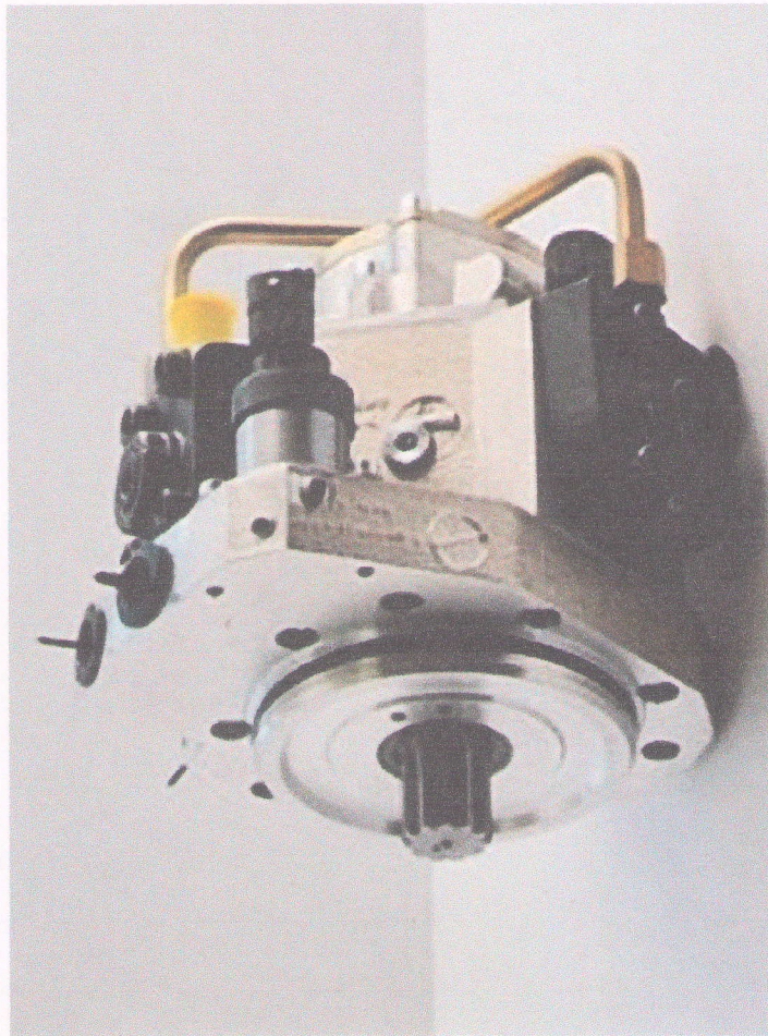
Рисунок 1 – ТНВД А-08-004-00-00-01
